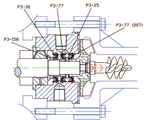
Vedação dupla
