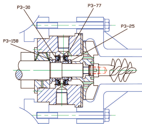
Vedação individual
